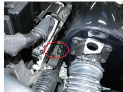
13. ビスCを使用してカーボンケースASSYを車両に固定します。
