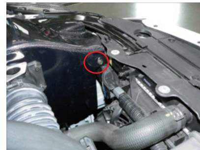
14. ビスBを使用してスTEE-BとカーボンケースASSYを固定します。
