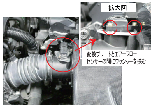
16. ビスFとワッシャーを使用してエアフローセンサーを取付けます。
