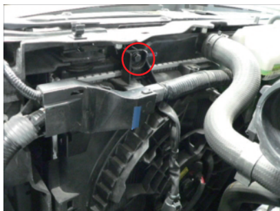
6. O印部のボルトを取外します。 ※取外した純正ボルトは使用しません。
