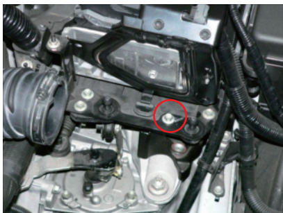
5. O印部のボルトを取外します。 ※取外した純正ボルトは使用しません。
