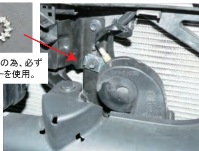
5.図を参考に、ホーンを図示の位置に移設します。移設に際しては、歯付きワッシャーをシュラウドパネルとホーンステーの間に挟み純正ボルトで取付けます。（ホーン移設後に動作確認を行ってください。）
