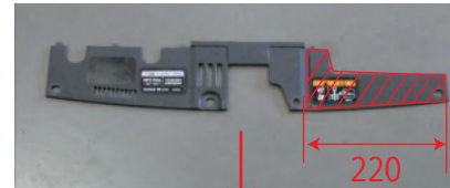
3.ホーン（LH）から取付けステーを一旦外し、表裏反転して取付けます。
