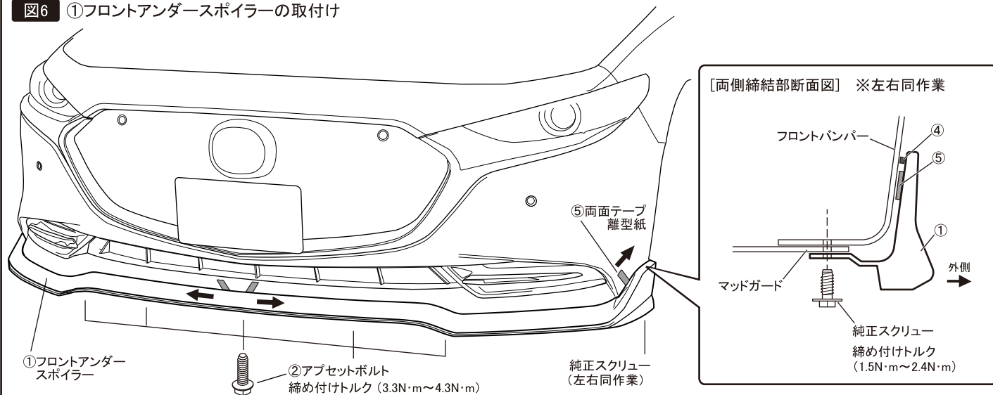
図6 ①フロントアンダースポイラーの取付け
