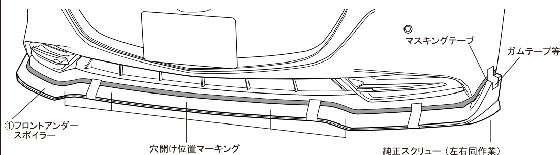
図2 ①フロントアンダースポイラーの仮当て
