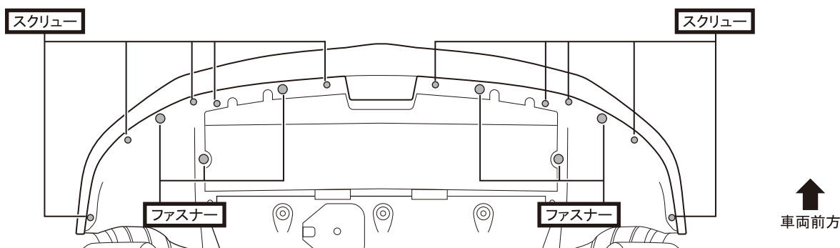
図1 純正スクリューと純正ファスナの取外し
