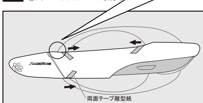
図3 ①ドアハンドルカバーの取付け
