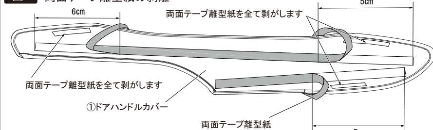
図1 両面テープ離型紙の剥離
