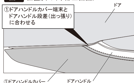
図2 位置決め(印部上面図)
